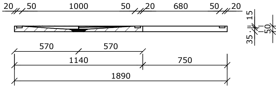
Schnitt A-A
